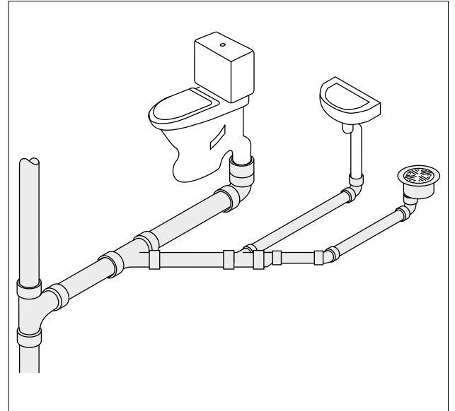
Kuva 65. Supistusyhteen asennus
