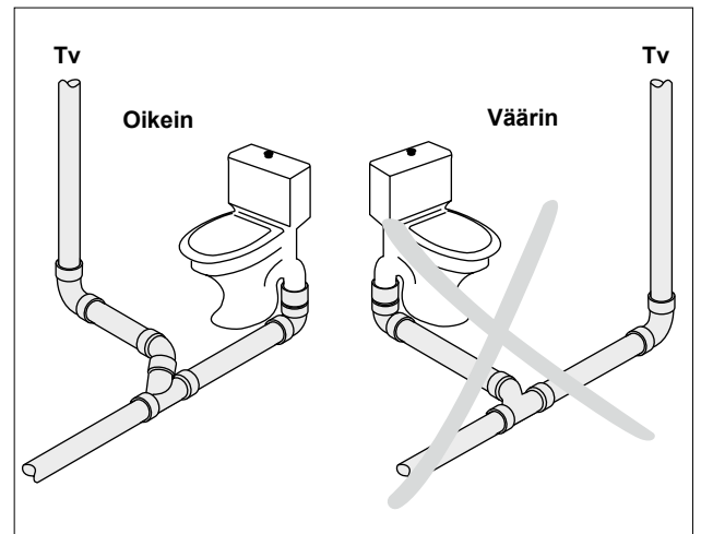
Kuva 66. Tuuletusviemärin liittäminen vaakakokojaviemäriin.
