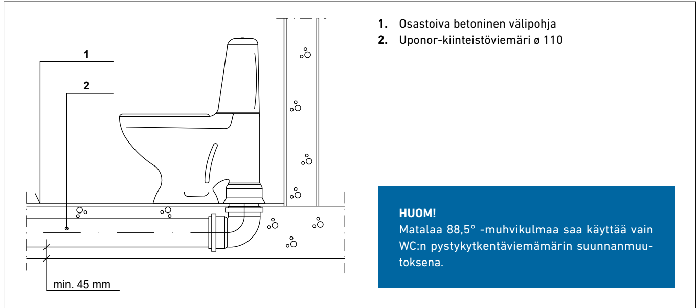
Kuva 54. WC-istuimen liittämisen viemäriin Uponor WC-mansetin ja matalan WC-muhvikulman avulla välipohjassa.
