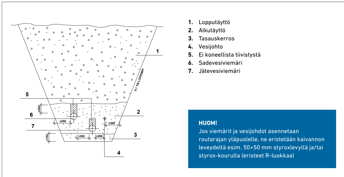
Kuva 44. Viemärikaivannon täytöt ja viemärien etäisyydet kaivannon reunoista sekä muista viemäreistä ja vesijohdoista.
