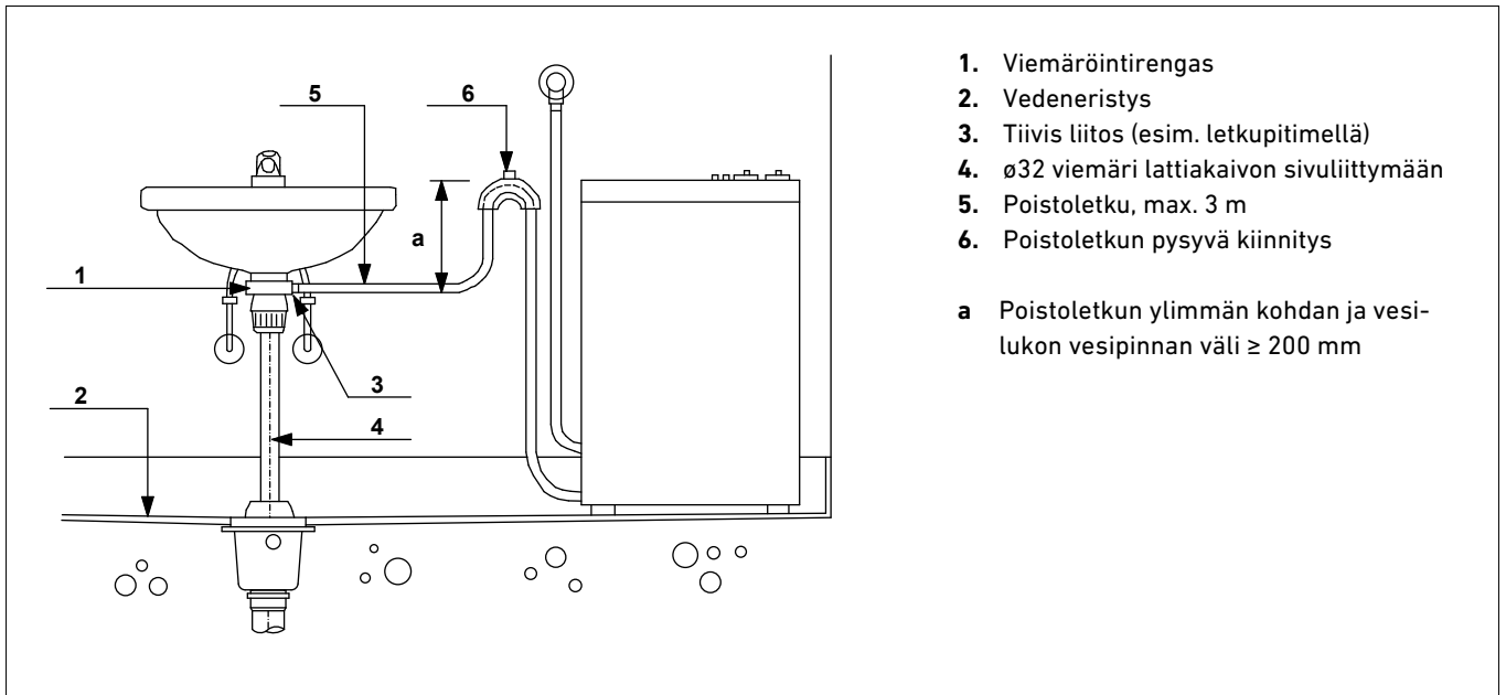
Kuva 69. Pesukoneen liittäminen viemäriverkostoon pesualtaan vesilukon yhteyteen asennetulla viemäröintirengaalla.
