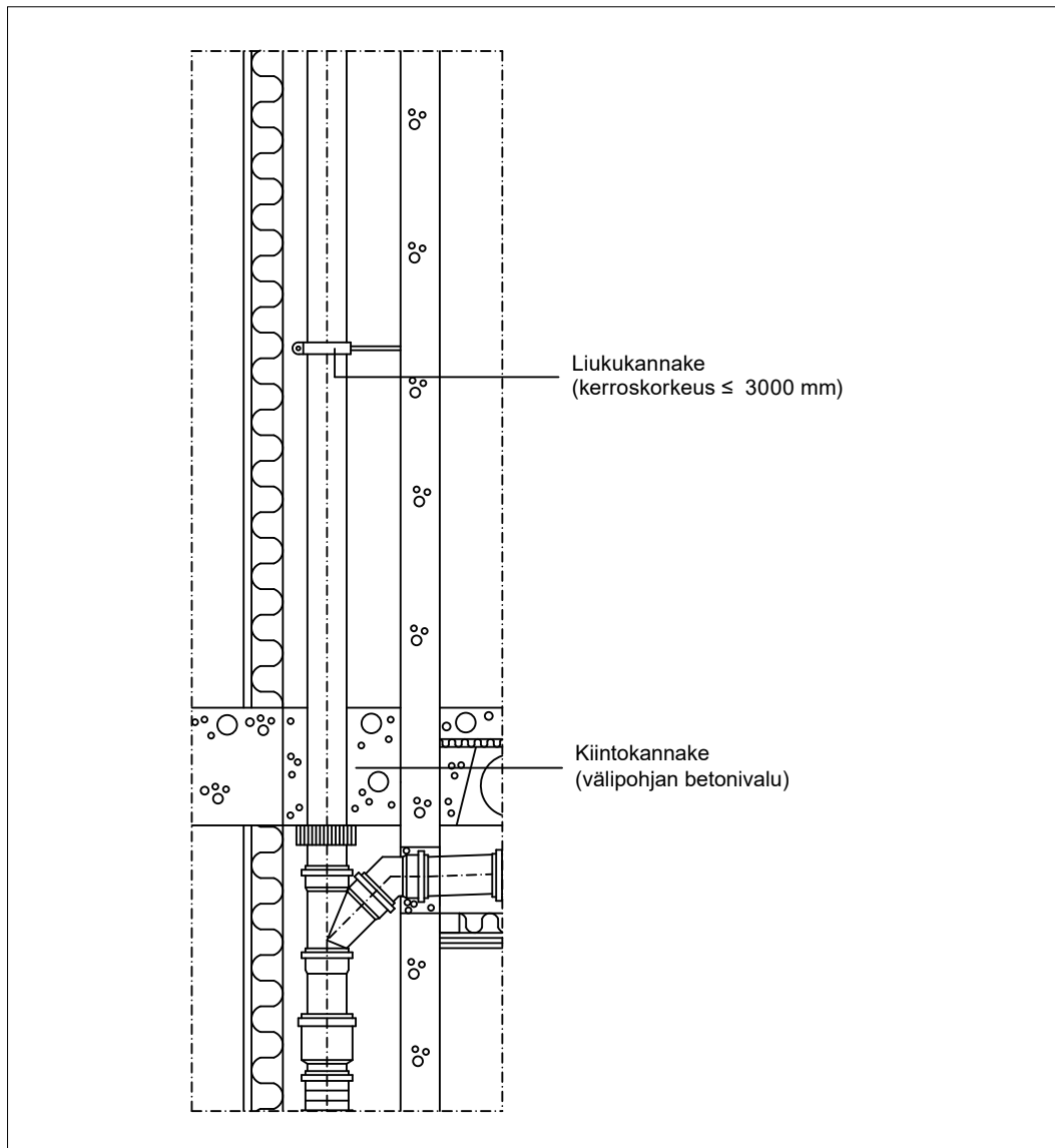
Kuva 43. Esimerkki pystyviemärin kannakoinnista.
