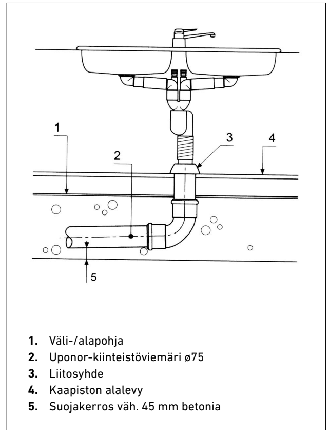
Kuva 59. Astianpesualtaan liittäminen viemäriin liitosyhteen avulla.
