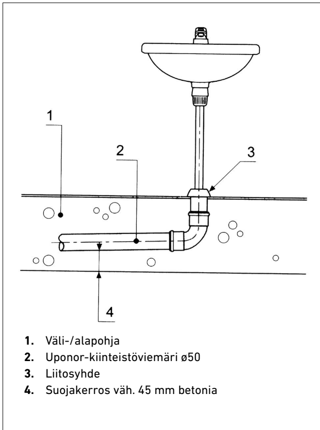
Kuva 58. Pesualtaan liittäminen viemäriin liitosyhteen avulla.
