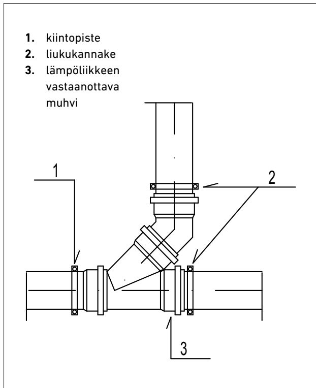
Kuva 41. Esimerkki vaakaviemärin haaroituksen kannakoinnista.
