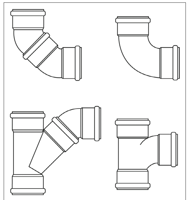
Kuva 35. Vaakaviemäriin liitos pystyviemäriin voidaan tehdä 45°-haarayhteen ja 45°-muhvikulman/kulmayhteen avulla tai poikkeustapauksessa käyttämällä 88,5°-loivakaarista muhvihaaraa/haarayhdettä. Vaakaviemäriin liitos vaakaviemäriin tehdään 45° haarayhteellä. Kyt-kentäviemäriin liitos vaakaviemäriin toteutetaan 45° haarayhteellä.
