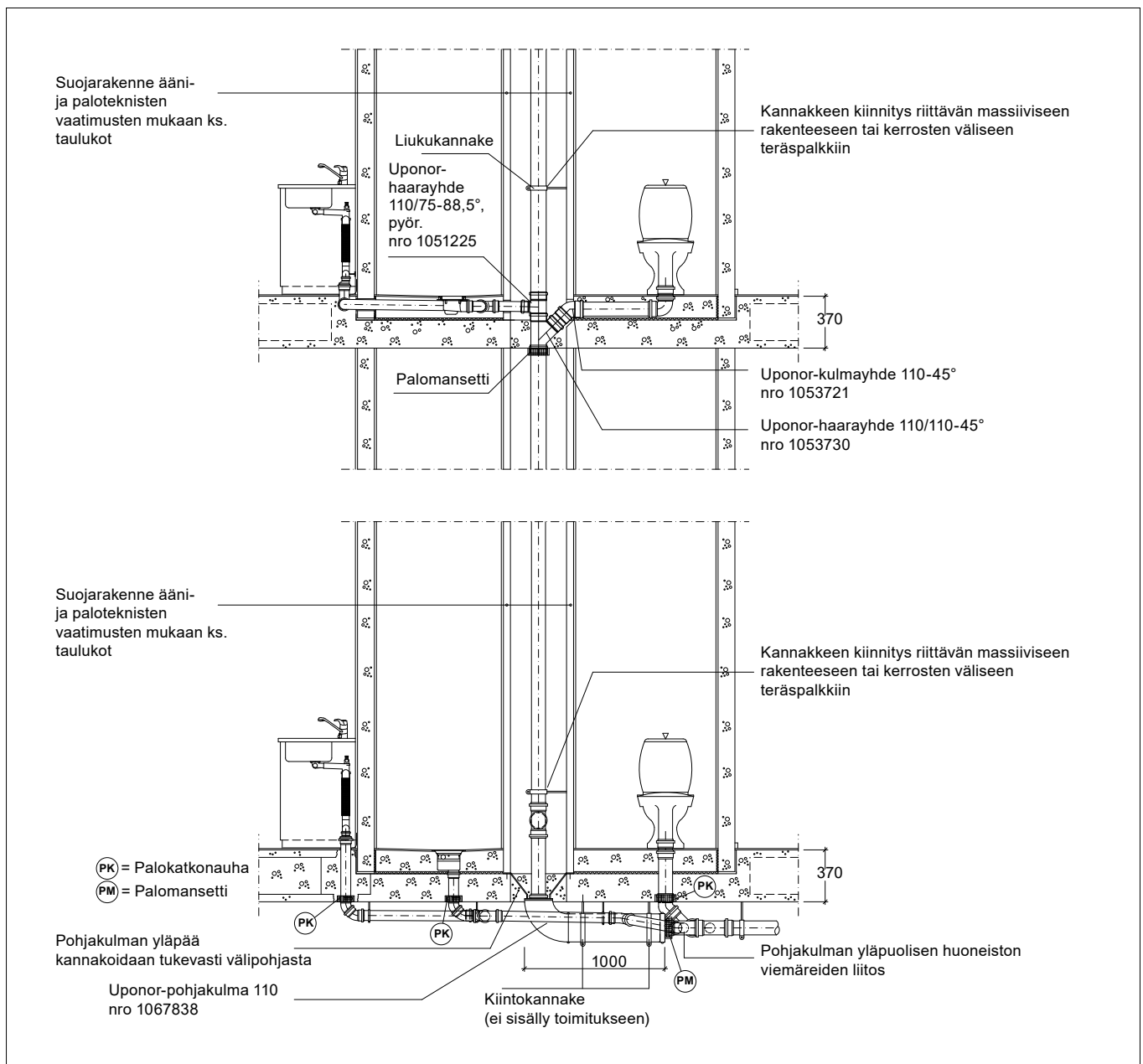
Kuva 33. Palomansetin ja/tai palokatkonauhan sijoitusperiaate Uponor-kiinteistöviemärien yhteydessä.
