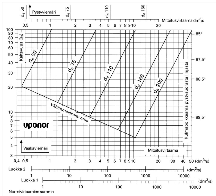
Kuva 37. Uponor-kokoojaviemärin mitoitusdiagrammi.
