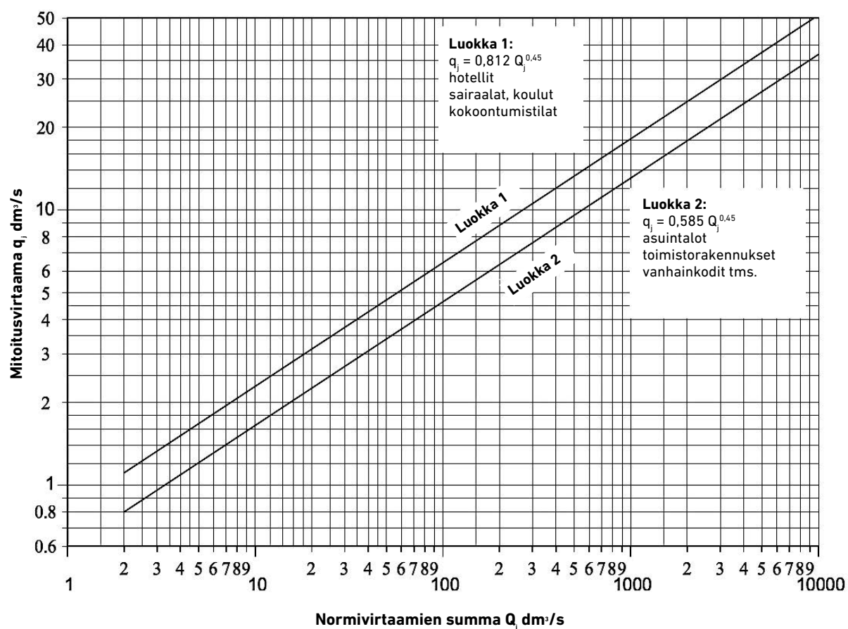
Taulukko 14. Viemärin mitoitusvirtaaman riippuvuus normivirtaamien summasta.
