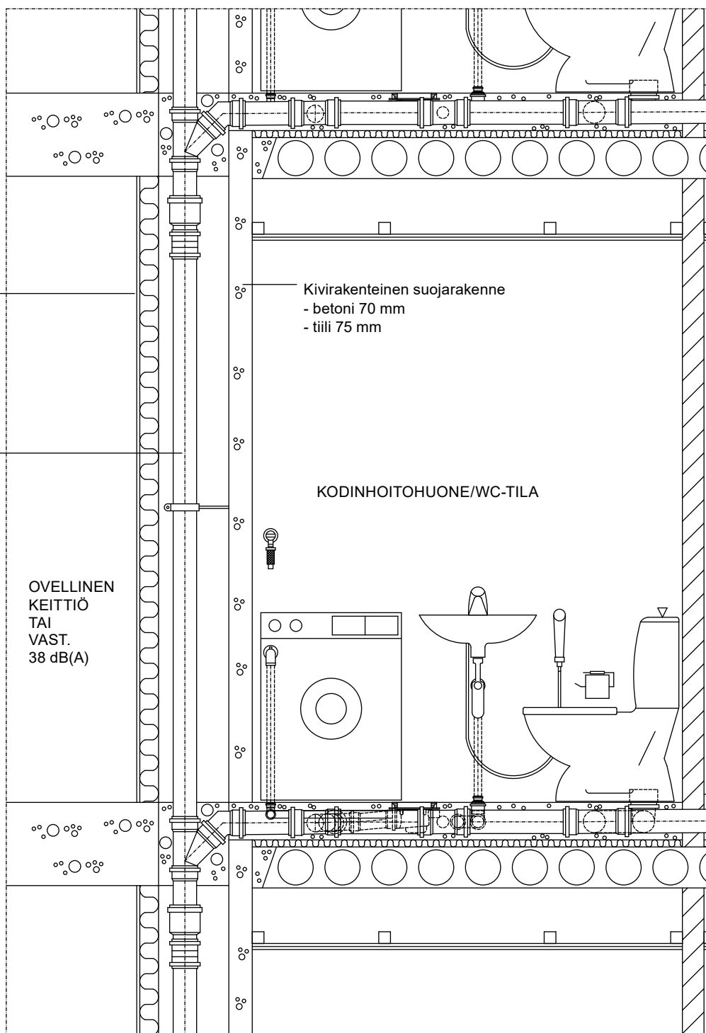
Kuva 11. Eristämättömän Uponor HTP -kiinteistöviemärin äänitekniset suojarakenteet pohjakulman kahden yläpuolisen (3. krs-) kerroksen yläpuolella, äänitasovaatimus 38 dB(A), EI 30.
