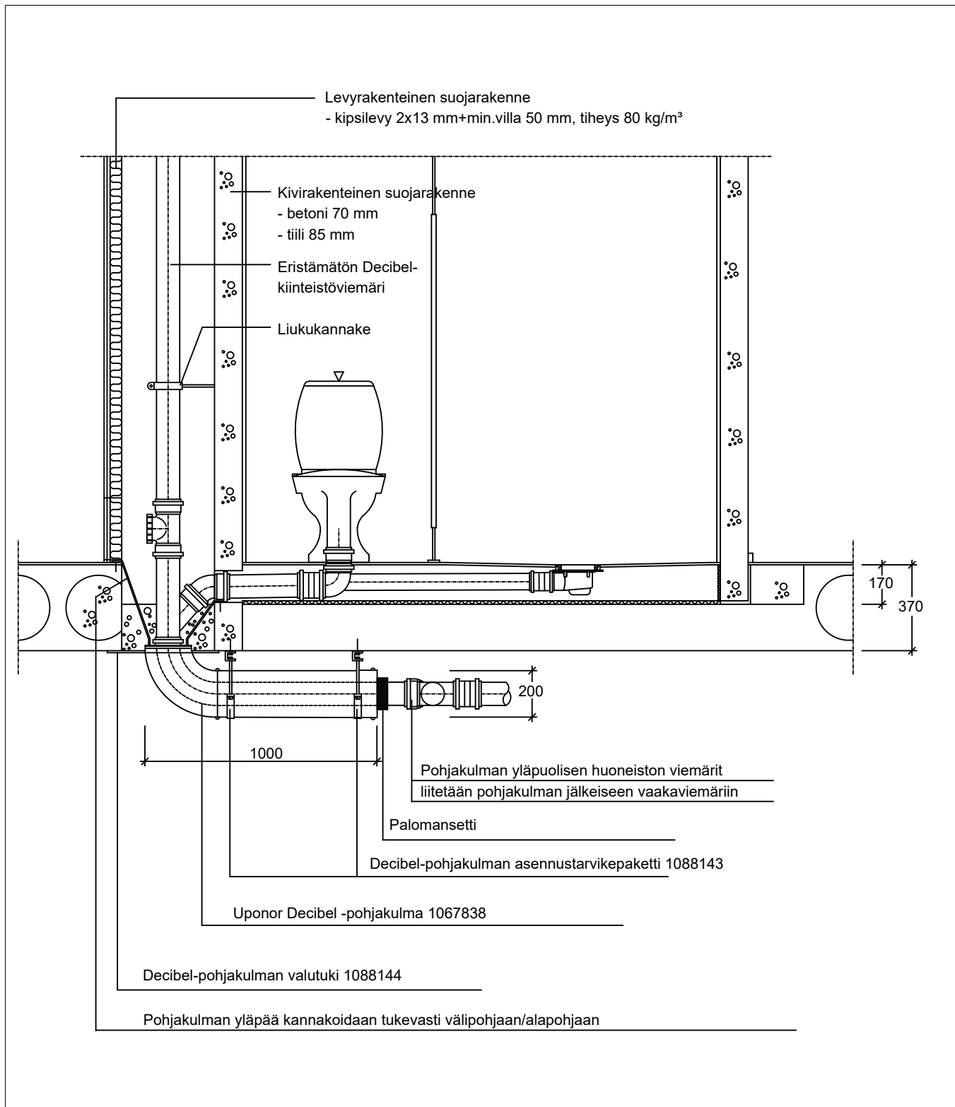
Kuva 22. Eristämättömän Uponor Decibel -kiinteistöviemärin äänitekniset suojarakenteet, äänitasovaatimus 28 dB(A). Pohjakulman yläpuolista huoneistoa palvelevia viemäriputkia ei liitetä pystykokoojaviemäriin, vaan ne johdetaan alapohjan alapuolelle ja liitetään äänenvaimentimen jälkeiseen vaakaviemäriin.
