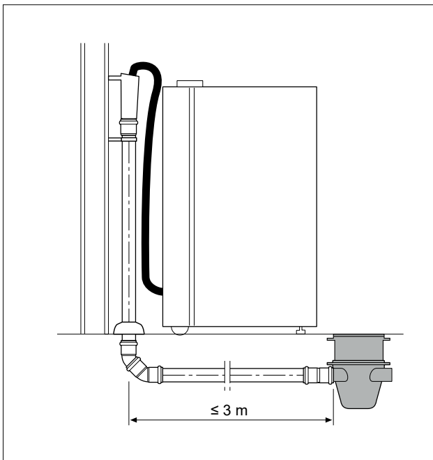
Kuva 63. Pesukoneen liittäminen viemäriverkostoon pesukonesuppilolla.
