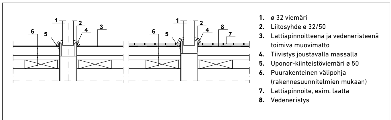
Kuva 68. Esimerkki kytkentäviemäriin läpiviennistä kostean tilan puurakenteisessa välipohjassa.
