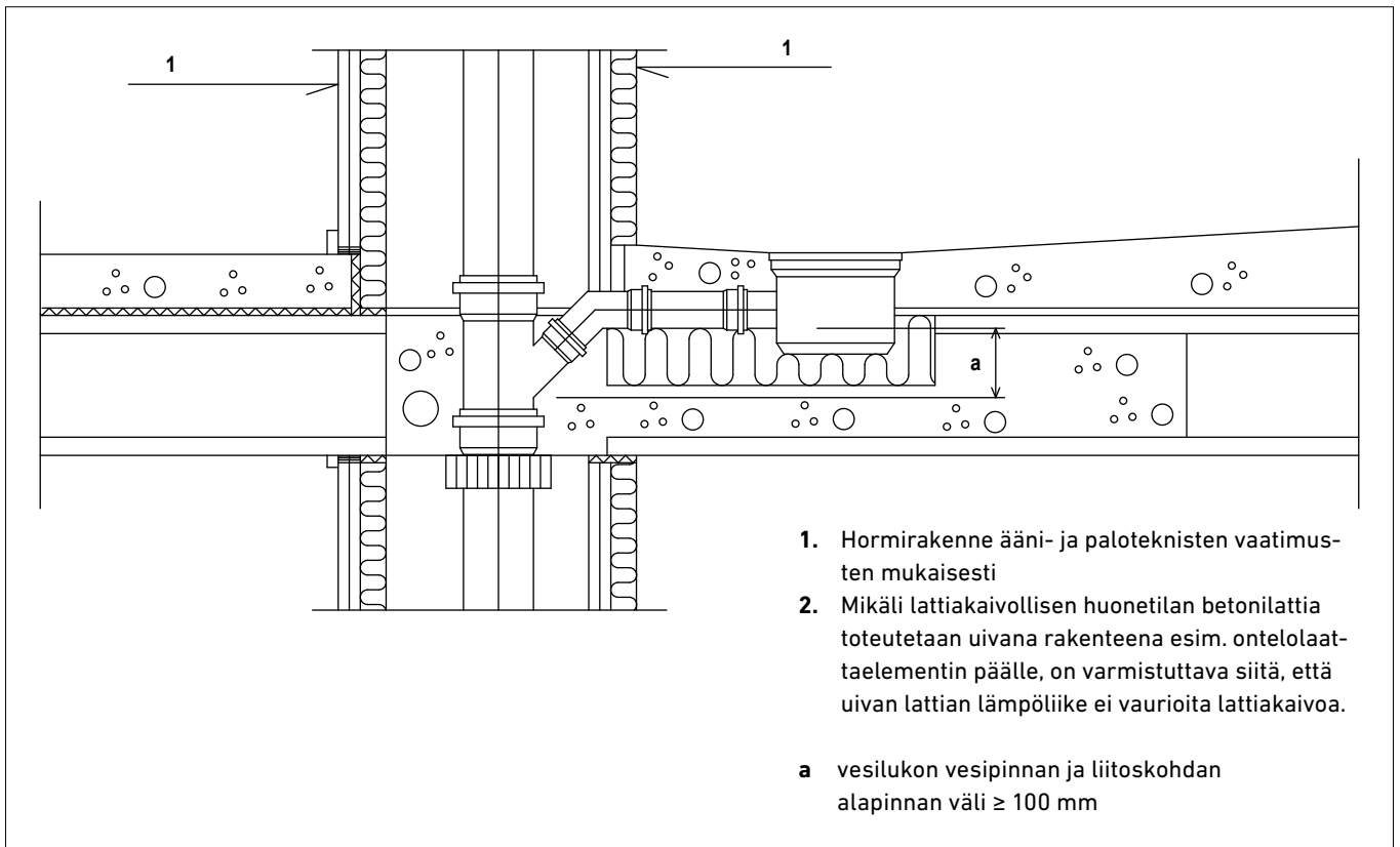
Kuva 60. Lattiakaivon kytkentäviemäriin liittäminen 45°-haarayhteellä pystykokojaviemäriin.
