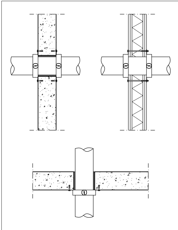
Kuva 71. Osastoivan rakenteen pintaan asennettava palomansetti seinä- ja lattiarakenteen läpivienneissä.
