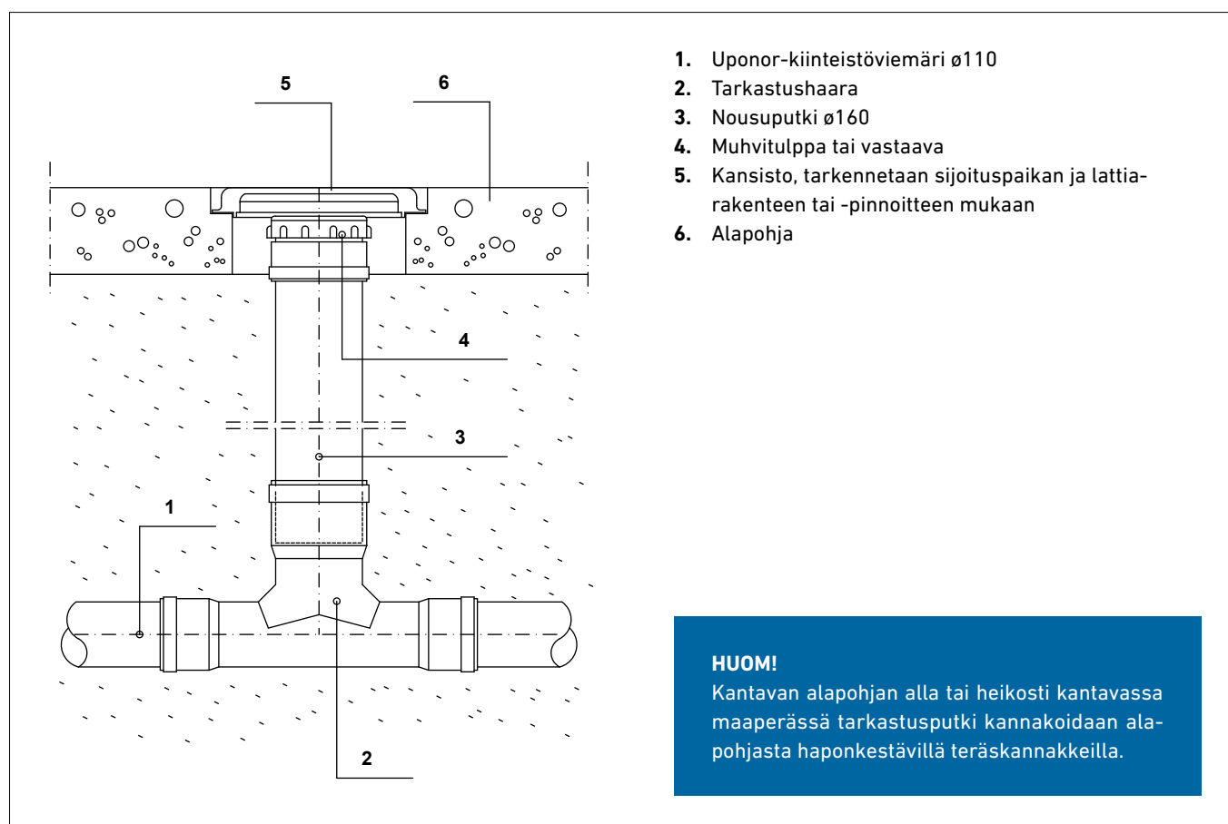
Kuva 73. Esimerkki rakennuksen sisäpuolisesta puhdistusluukusta ja tarkastusputkesta.
