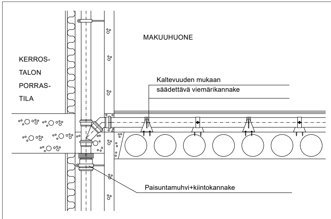
Kuva 42. Vaakaviemärin kannakointi ns. asennuslattiasa.
