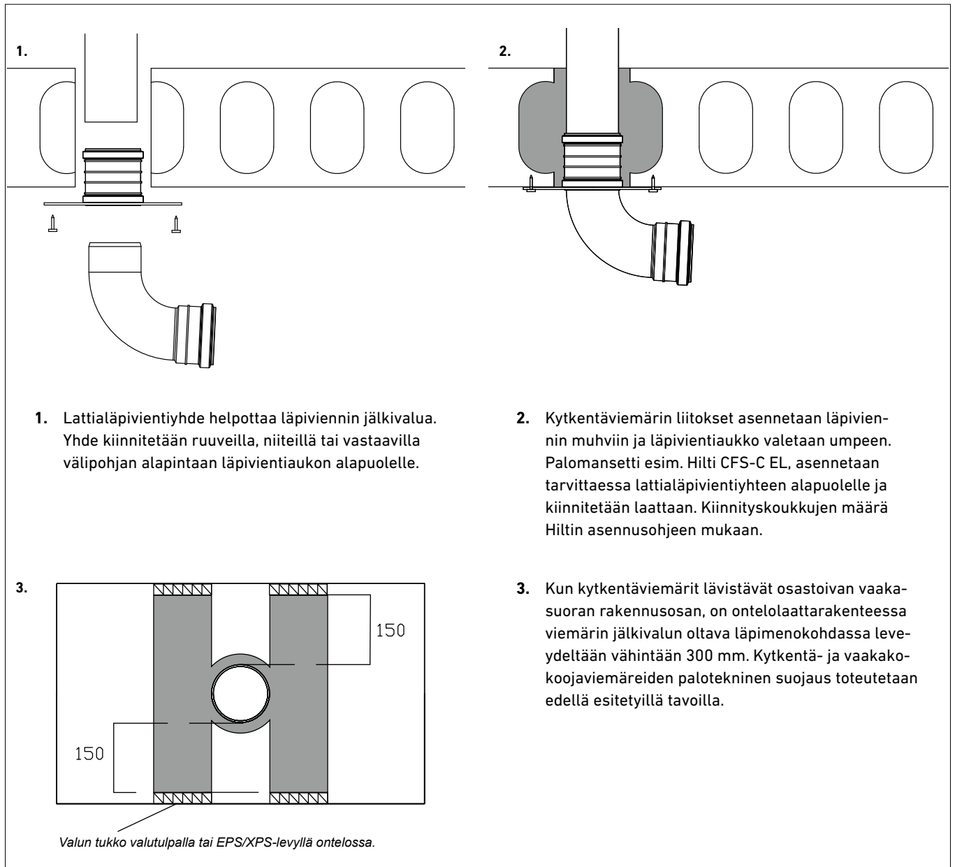
Kuva 34. Lattialäpiviennit.
