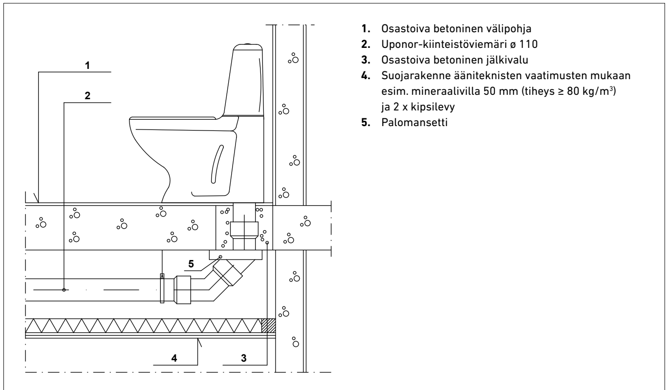
Kuva 55. WC-istuimen liittämisen viemäriin Uponor WC-mansetin ja matalan WC-muhvikulman avulla välipohjassa.
