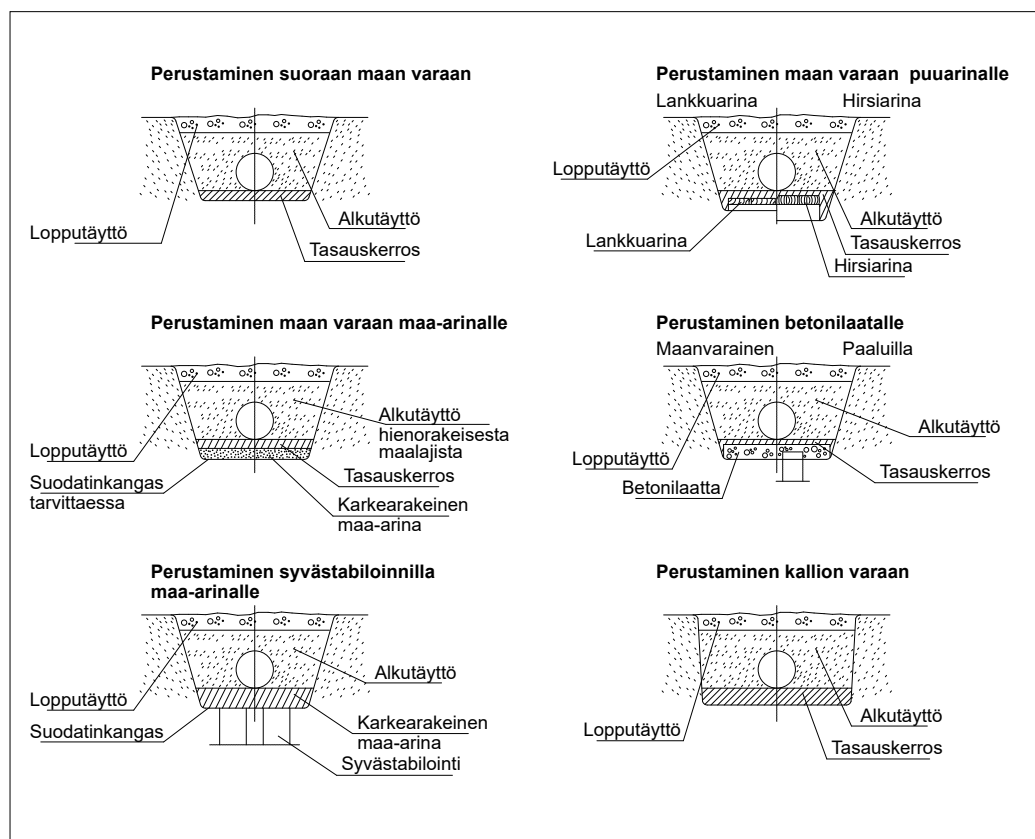
Kuva 45. Putkiarina. Arina voidaan tehdä sinkitystä profiliteräslevystä, betonista tai sopivasta maa-aines-kerroksesta.
