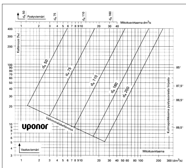
Kuva 39. Mitoitusdiagrammi Uponor-sadevesiviemäreille.
