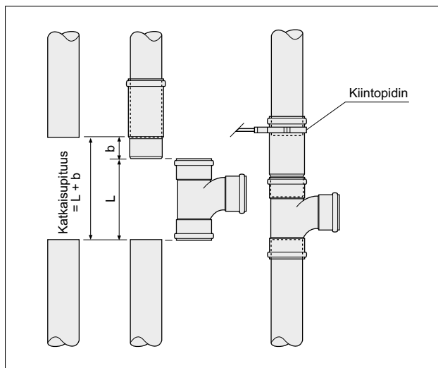
Kuva 50. Haaroitus muhvihaaran ja liitos-/paisuntayhteen avulla.
