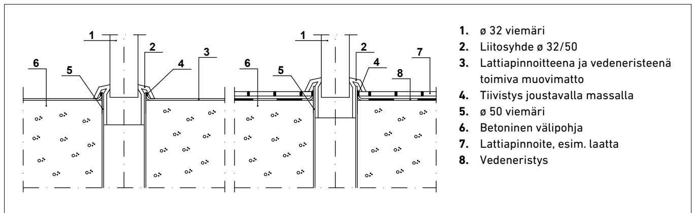
Kuva 67. Esimerkki kytkentäviemäriin läpiviennistä kostean tilan betonirakenteisessa välipohjassa.
