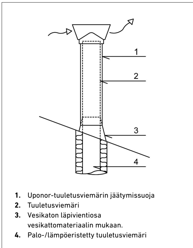
Kuva 72. Uponor-tuuletusviemärin jäätymissuoja asennettuna tuuletusviemärin vesikaton yläpuolisen osan päälle.
