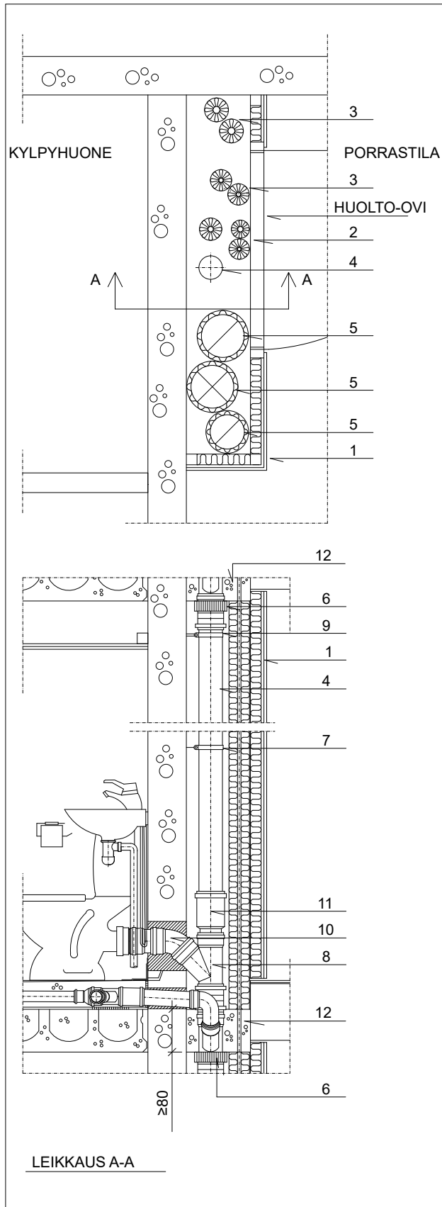
Kuva 16. Esimerkki levyrakenteisesta seinärakenteesta eristämättömän Uponor Decibel -kiinteistöviemärin yhteydessä. Äänitasovaatimus 33 dB(A). EI 30.
