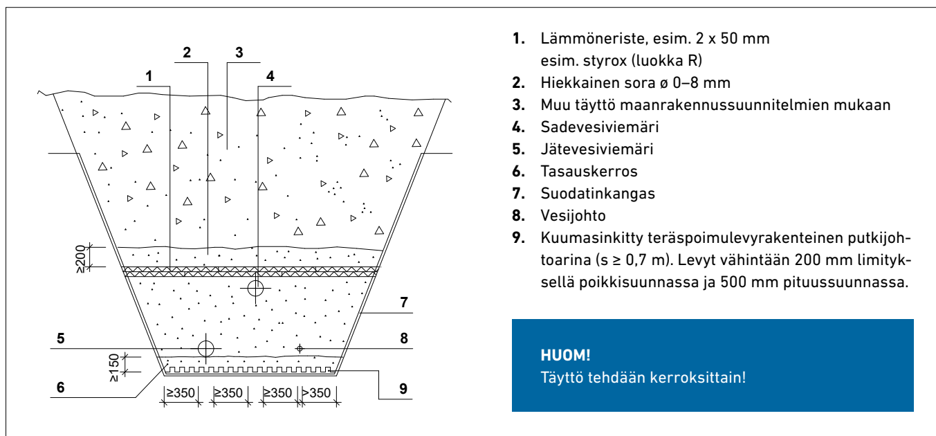
Kuva 45. Putkiarina. Arina voidaan tehdä sinkitystä profiliteräslevystä, betonista tai sopivasta maa-aines-kerroksesta.
