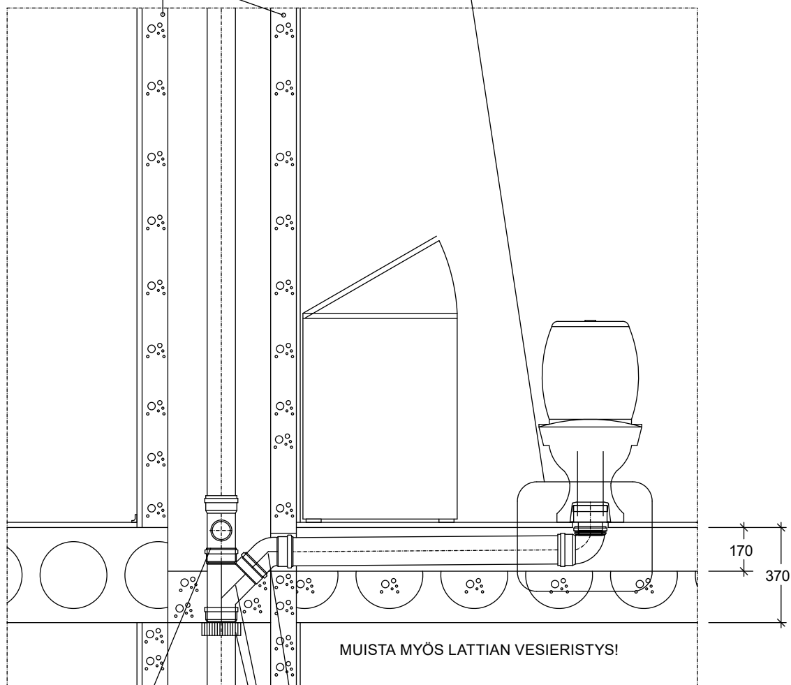
Uponor-haarayhde 110/75-45° nro 1053729
