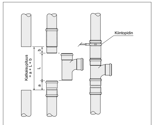
Kuva 51. Haaroitus haarayhteen, kaksoismuhvin ja liitos-/paisuntayhteen avulla.
