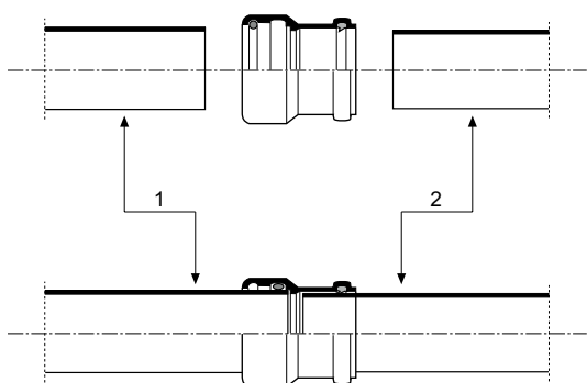
Kuva 52. Valurauta- ja Uponor-viemärien liittäminen jatkoysteellä, jossa on kumitiiviste molemmille putkille (koot 75/70 ja 110/100 putkille).
