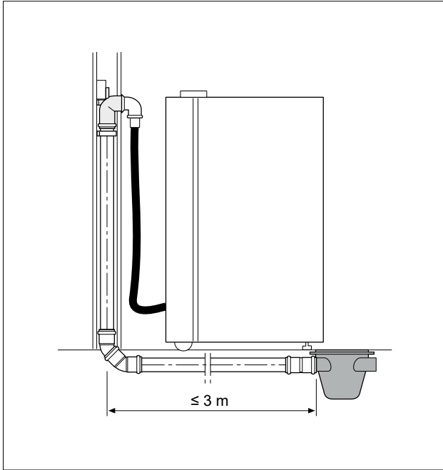
Kuva 61. Pesukoneen liittäminen viemäriverkostoon viemärintikulmalla ja kulmaliittimellä.
