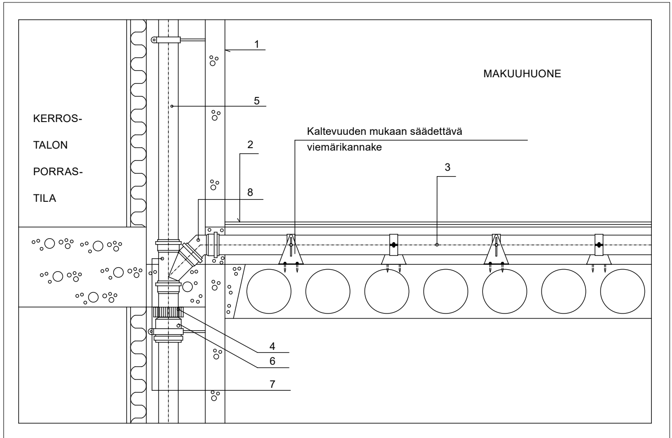
Kuva 21. Esimerkki kytkentä- ja vaakakokoojaviemärien asennuksesta ns. kerroslattian yhteydessä. Palomansetillä saavutetaan vaadittava palo-osastointiluokka.
