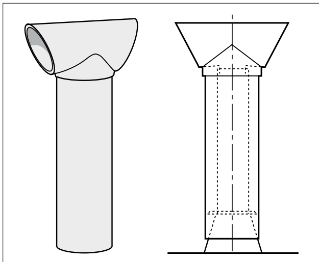
Kuva 38. Tuuletusviemärin jäätymissuoja tuuletusviemäriin asennettuna.
