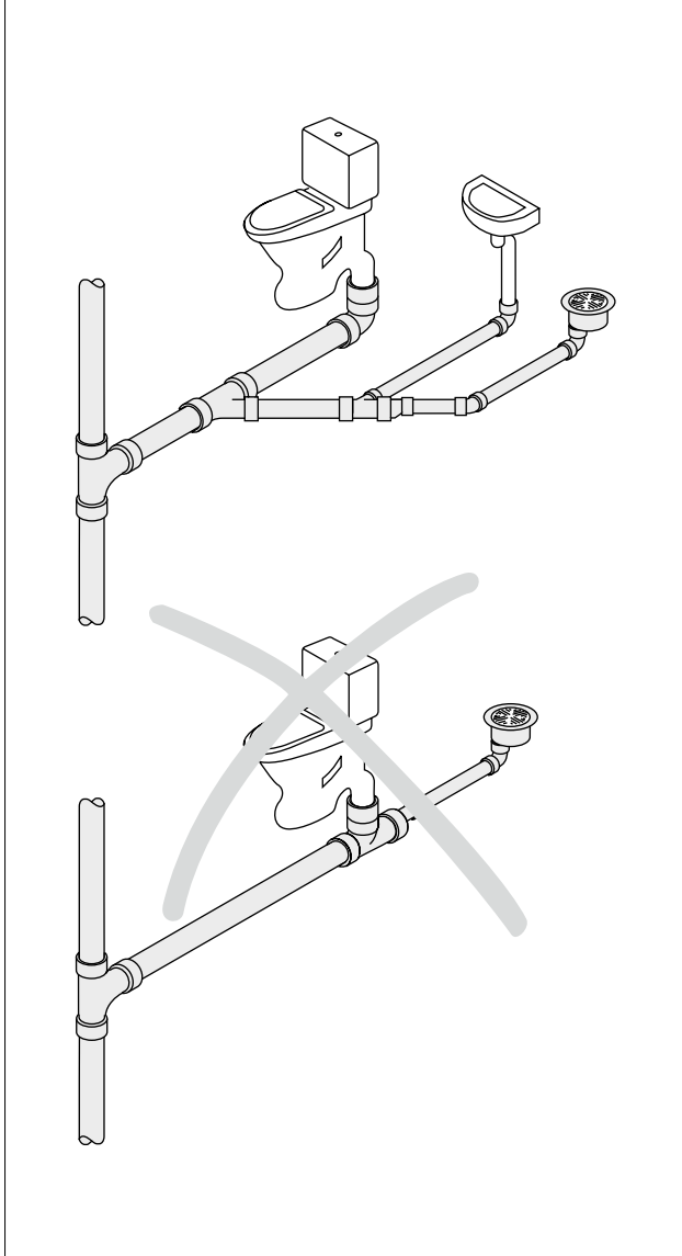
Kuva 64. Kytkentäviemärin liittäminen WC-istuimen tuulettamattomaan viemäriin.
