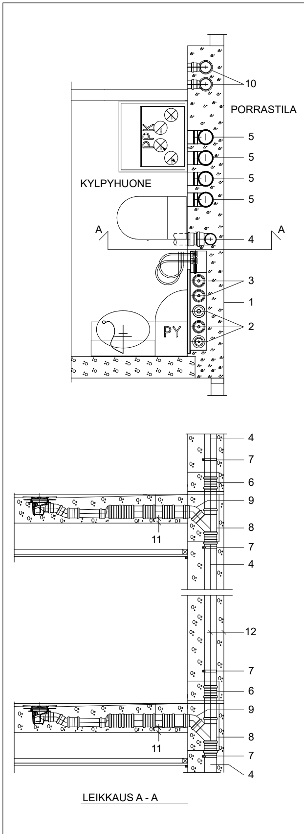
Kuva 15. Esimerkki Parman betonisesta tekniikkaseinäelementistä Decibel-kiinteistöviemärin yhteydessä, äänitasovaatimus 33 dB(A). EI 60.
