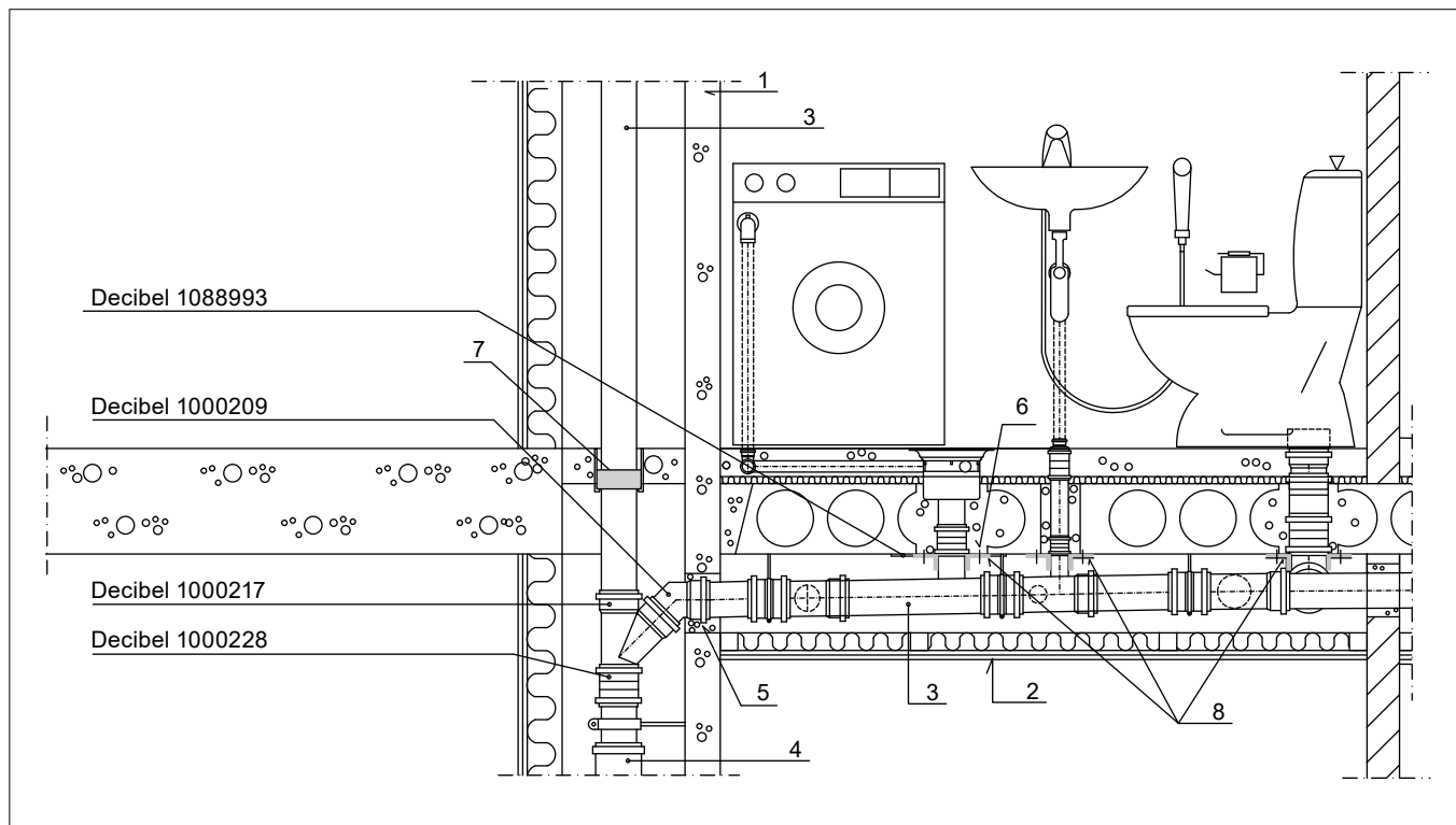
19. Esimerkki Uponor Decibel -kiinteistöviemärin asennuksesta alasasketun kattorakenteen yläpuolelle.
