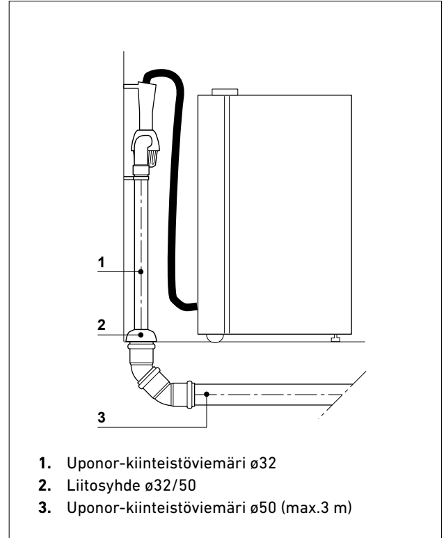
Kuva 62. Pesukoneen liittäminen viemäriverkostoon vesilukollisella pesukonesuppilolla.
