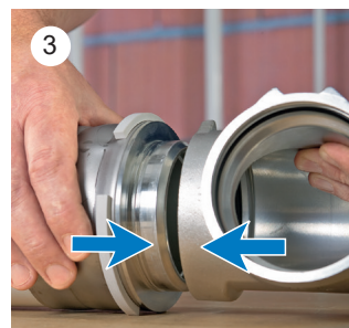
Kuva 1. Asenna viistetty komposiittiputki Uponor RS-liitinjärjestelmän puristuspäähän.
