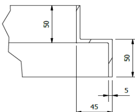
Rammeprofil:
