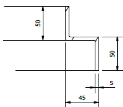
Rammeprofil:
