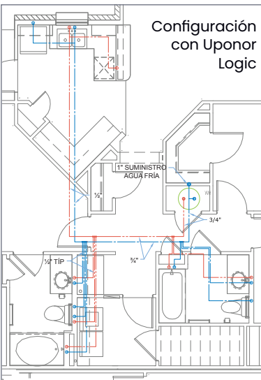
Figura 5-1: Configuración con Uponor Logic
