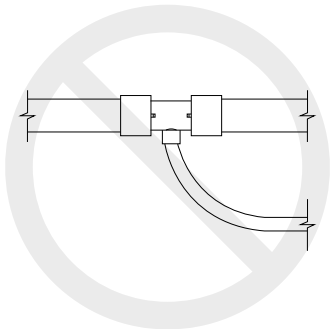
Figura 6-3: Curva incorrecta
