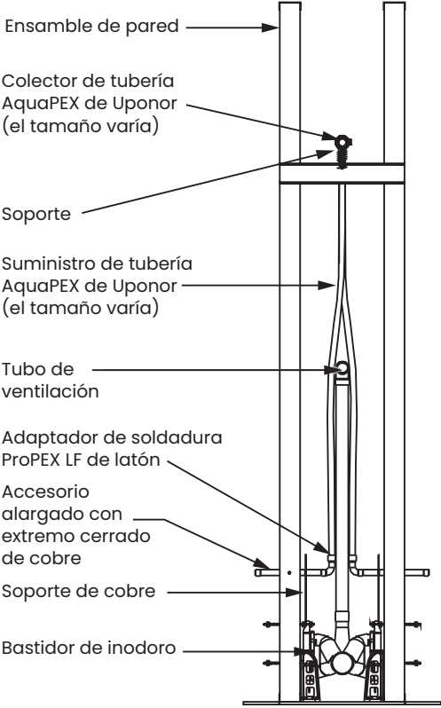
Figura 5-5: Imagen de la sección del banco del dispositivo
