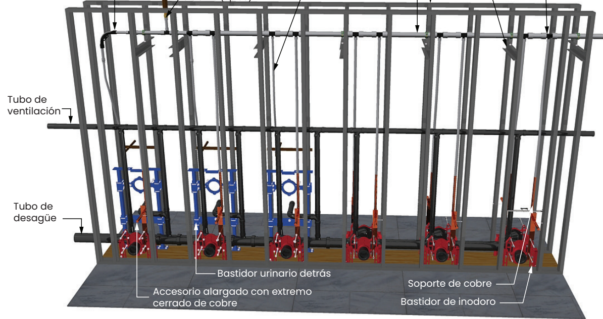
Figura 5-6: Imagen de la elevación del banco del dispositivo
