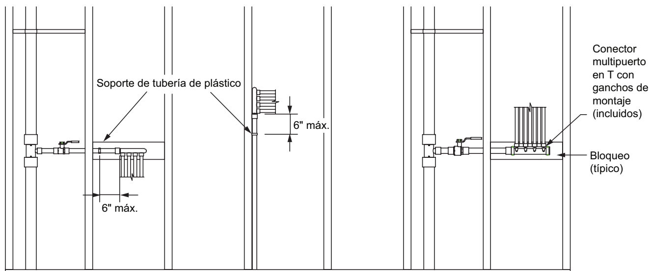
Figura 6-9: Soportes en la pared para conectores multipuerto en T
