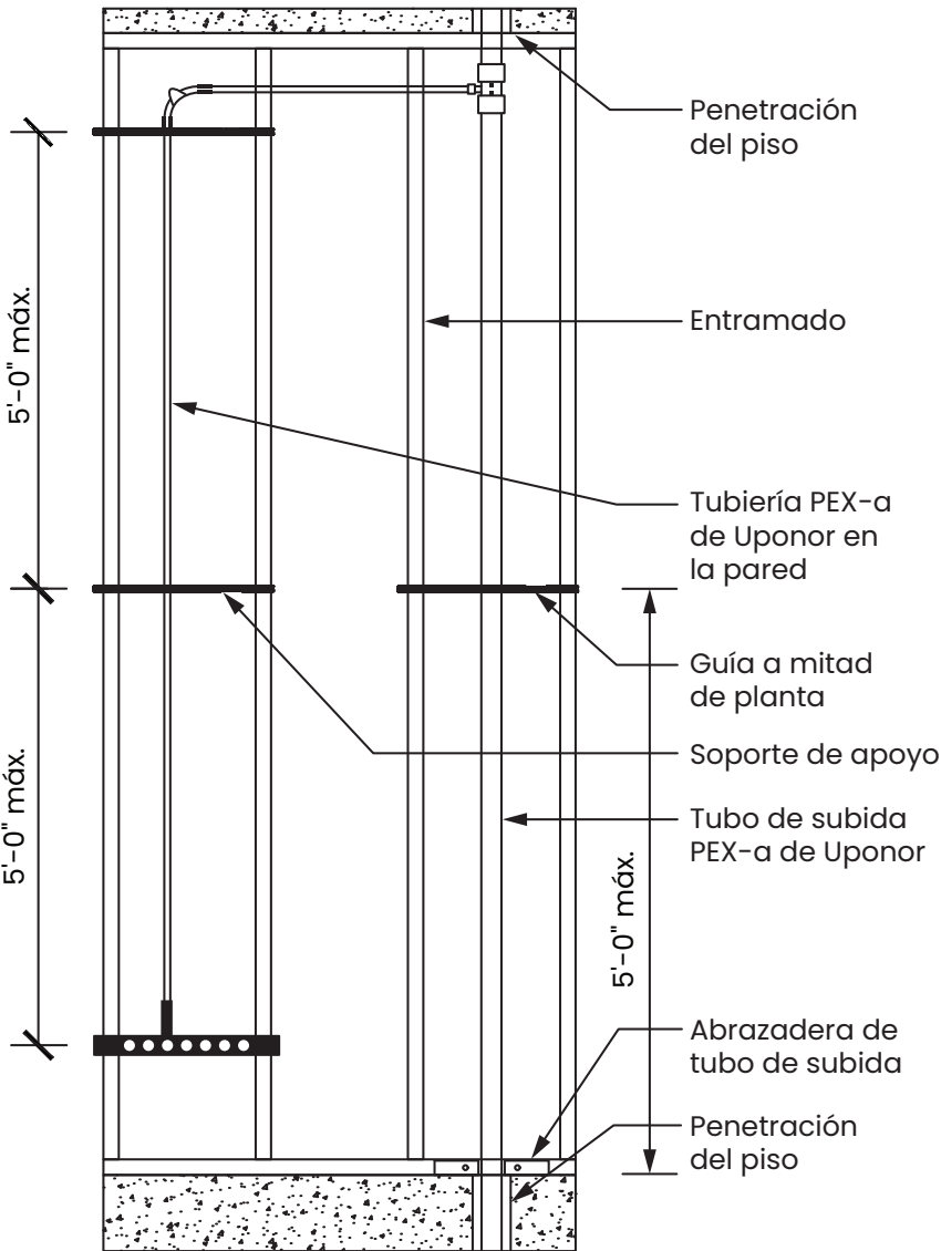
Figura 6-16: Tubería en la pared frente a tubos de subida
