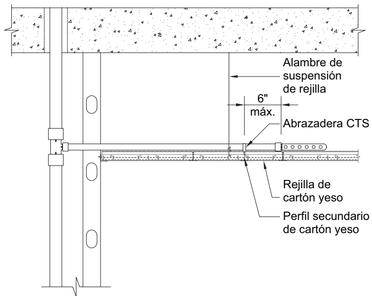
Figura 6-13: Apoyando a conectores multipuerto en T en rejilla de tabla roca
