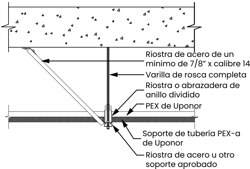
Figura 6-14: Punto fijo
