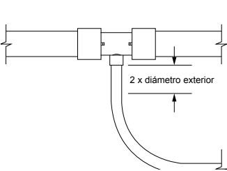
Figura 6-2: Curva correcta
