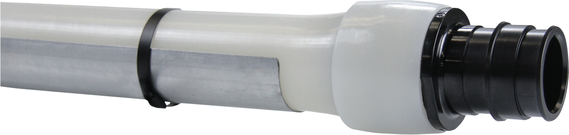
Figura 6-7: Soporte de tubería PEX-a de Uponor con flejado de nilón
