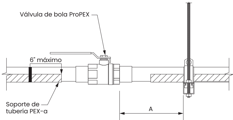
Figura 6-4: Apoyar a válvulas de bola de 1¼" a 2"
