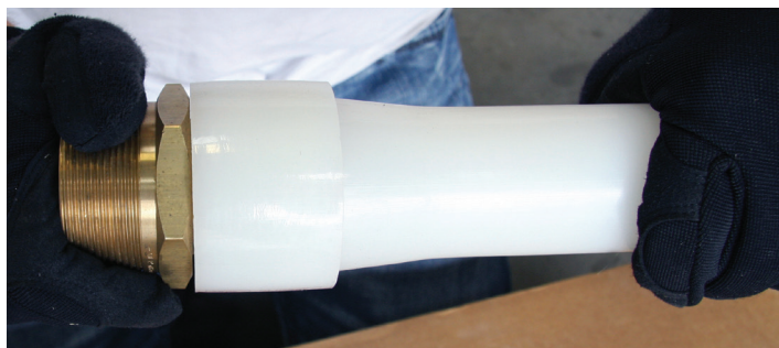
Figura 2-29: Accesorio ProPEX de latón conectado al tubo
