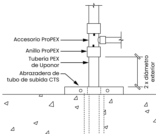
Figura 6-20: Ejemplo de distancia de abrazaderas
