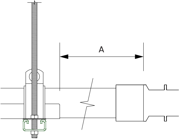
Figura 6-6: Distancia mínima al accesorio
