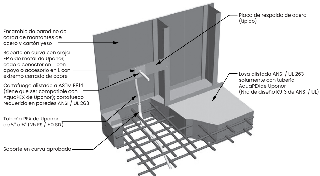
Figura 3-9: Detalle de dispositivo (EE. UU.)
