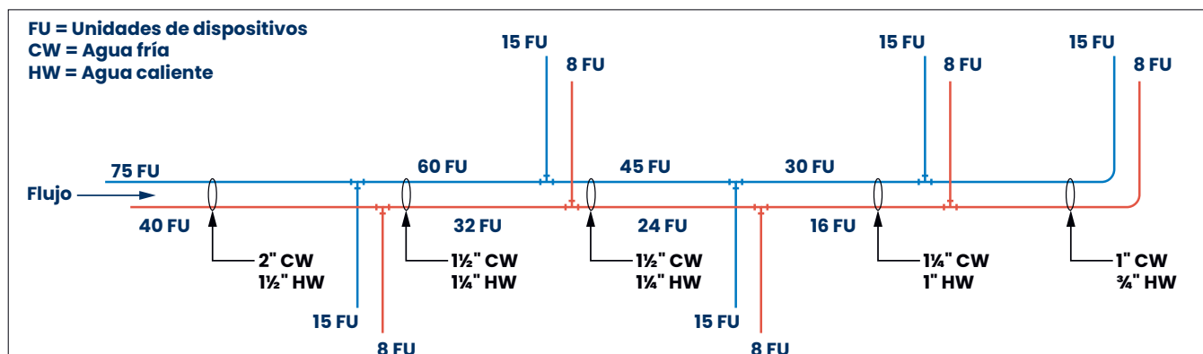
Figura 5-10: Utilice el cuadro de cantidad de agua en el diseño de la plomería
