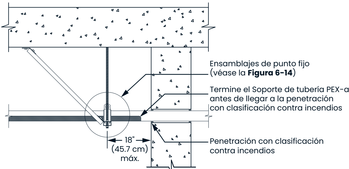
Figura 6-15: Puntos fijos cerca de una penetración con clasificación contra incendios (horizontal)
