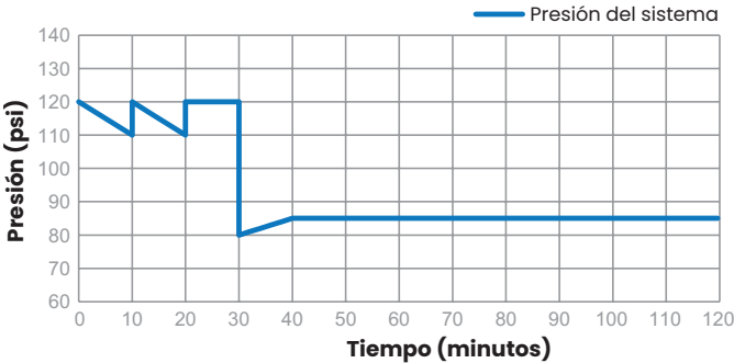
Figura 6-2: Gráfico de prueba de presión
