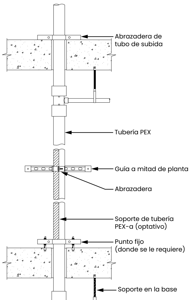
Figura 6-19: Detalle de tubo de subida PEX
