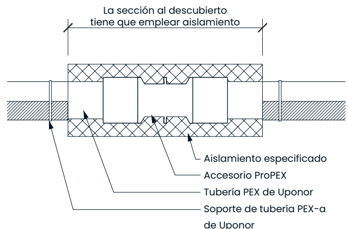
Figura 3-20: Instalaciones de Soporte de tubería PEX-a en aplicaciones ASTM E84
