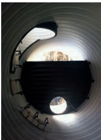
Wnętrze retencyjnego kanału ściekowego z przegradą piętrzącą wykonaną z PE-HD
