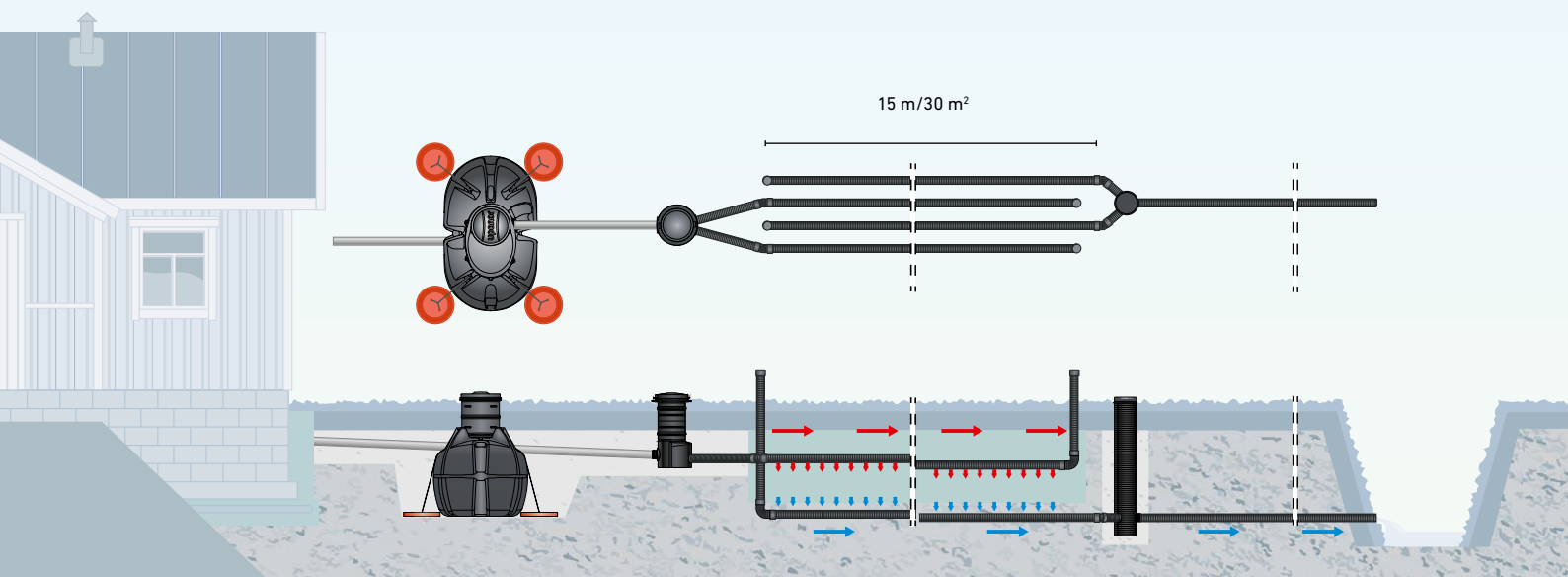
Uponor-maasuodattamo 2 m 3
