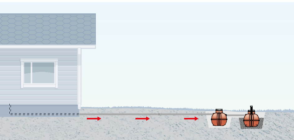
Saunasta pesuvedet johdetaan saunakaivoon ja kaivosta maaperään puhdistumaan. Mökkikaivo erottelee astianpesuvesistä kiinteät aineet sekä rasvan. Selkeytynyt vesi johdetaan eteenpäin saunakaivoon imeytettäväksi.
