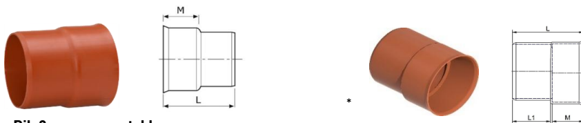
Ultra Rib 2 overgangsstykke Fra glat muffe til Ultra Rib 2-spidsende
