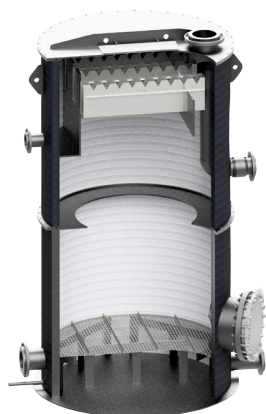
Alkaliseringsstank
