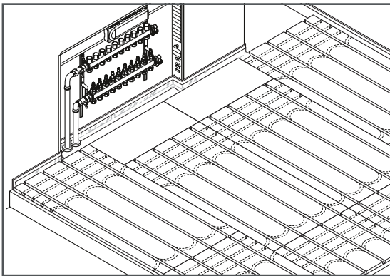
1. Asenna Siccus-paneelit.
