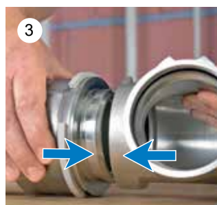
Kuva 1. Asenna viistetty komposiittiputki Uponor RS-liitinjärjestelmän puristuspäähän.
