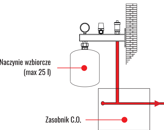
Grupa bezpieczeństwa do instalacji C.O.
