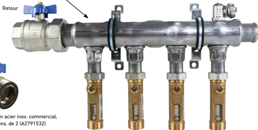
Robinet d'isolement à bille pour collecteur en acier inoxydable commercial (A2791010)
