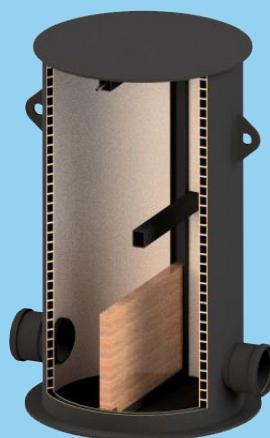
Nivåregleringsbrunn
