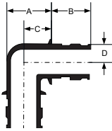
EP elbow
