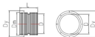
Ingjutningsmuffar Ø 175 – Ø 500.
