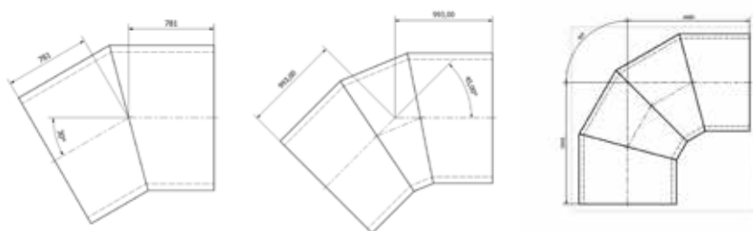
Böjar Ø 1200-2000
