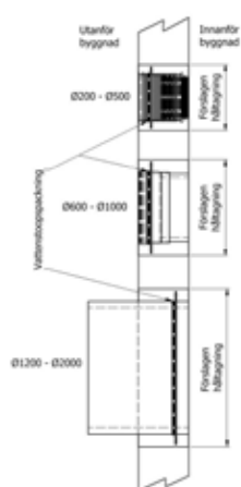
Skissen visar måttsett snitt i vägg med ingjutna muffar.
