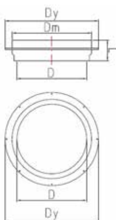
Ingjutningsmuffar Ø 600 – Ø 2500.
