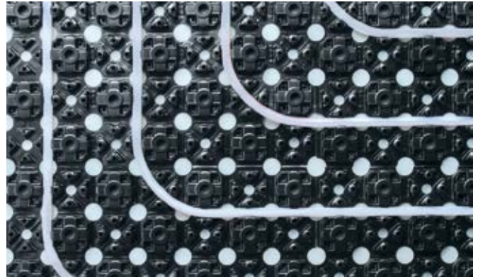
Ugradnja Uponor PE-Xa cijevi pod kutom od 90°
